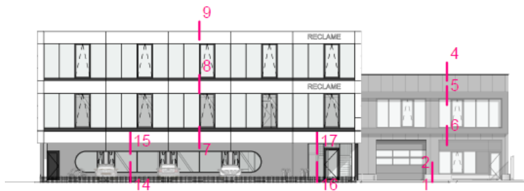
VOORGEVEL (NOORD)
